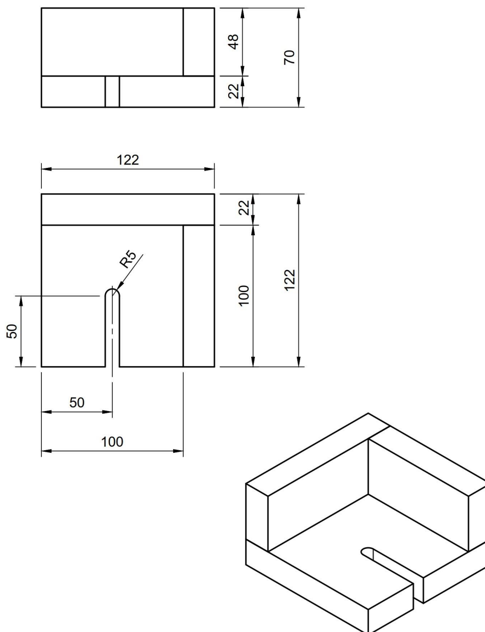
Рисунок 33 – Правая поддержка стационарного маяка
