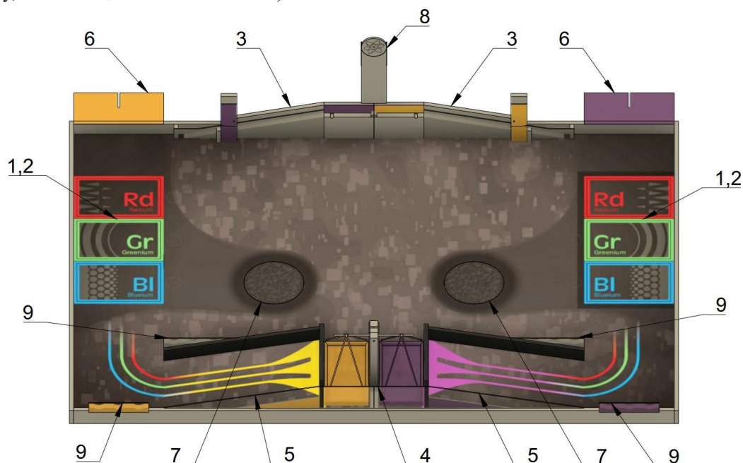
Рисунок 4 – Детальный вид Игрового поля
