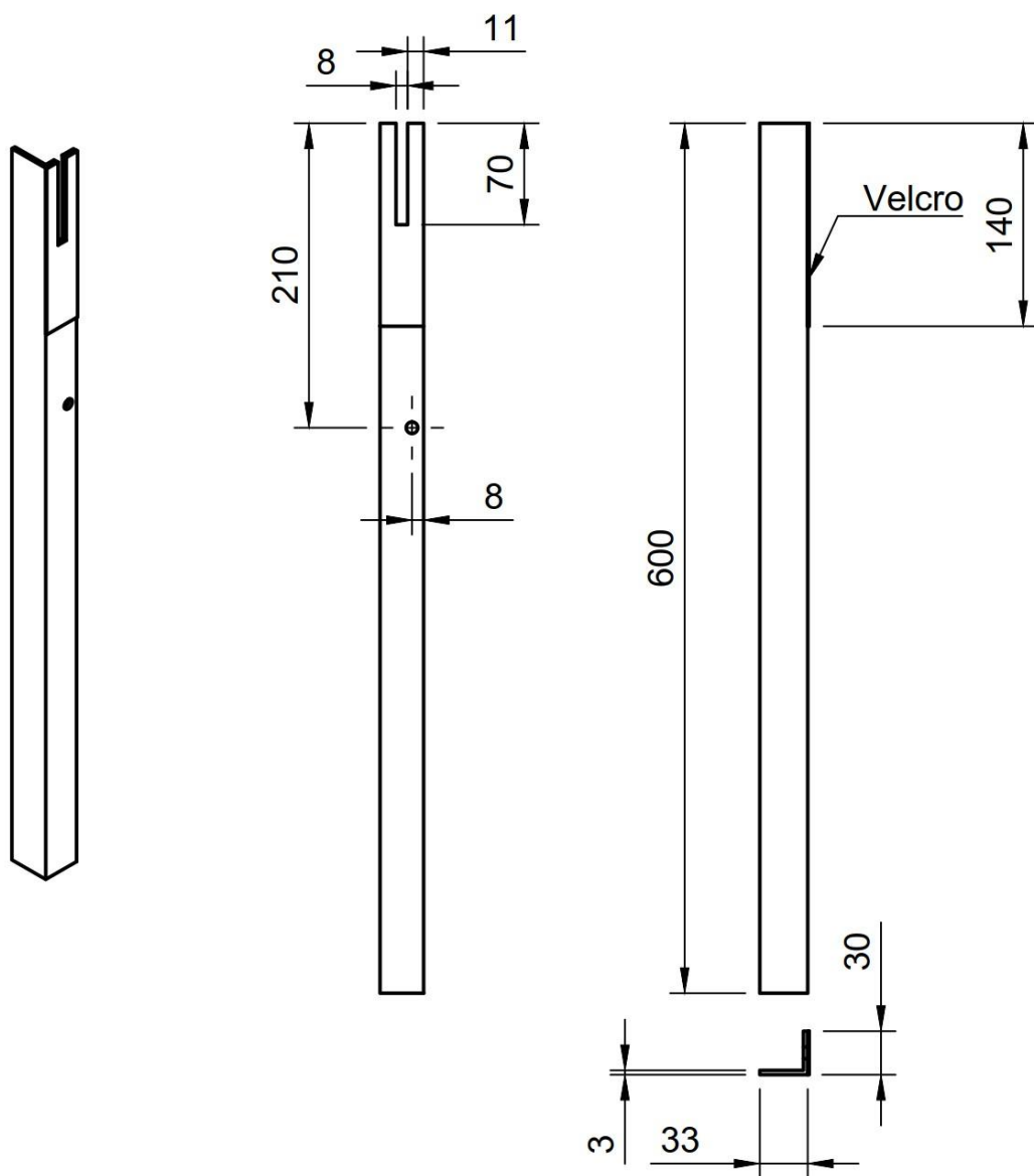
Рисунок 28 – Мачта эксперимента (прав)
