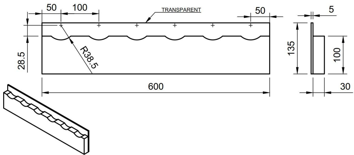
Рисунок 30 – Большой распределитель атомов
