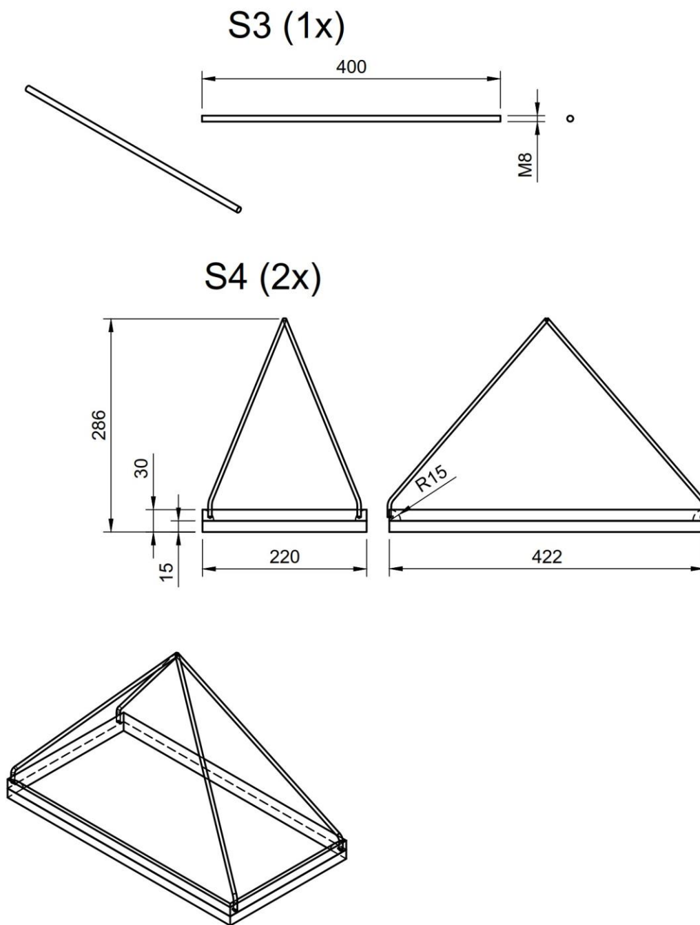
Рисунок 16 – Весы – детализированный вид 2
