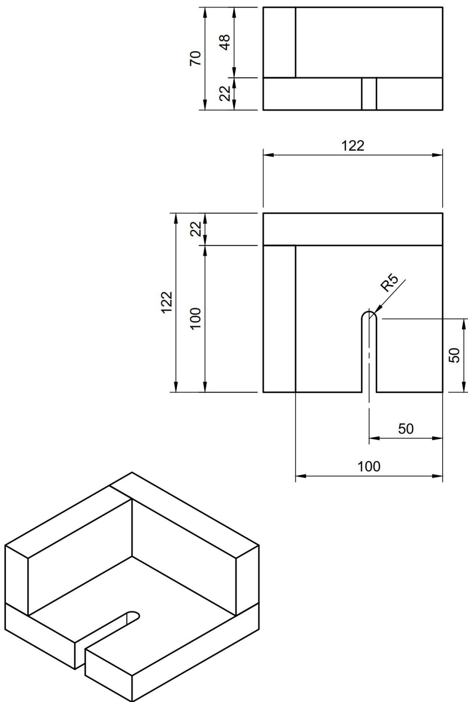
Рисунок 32 – Левая поддержка стационарного маяка
